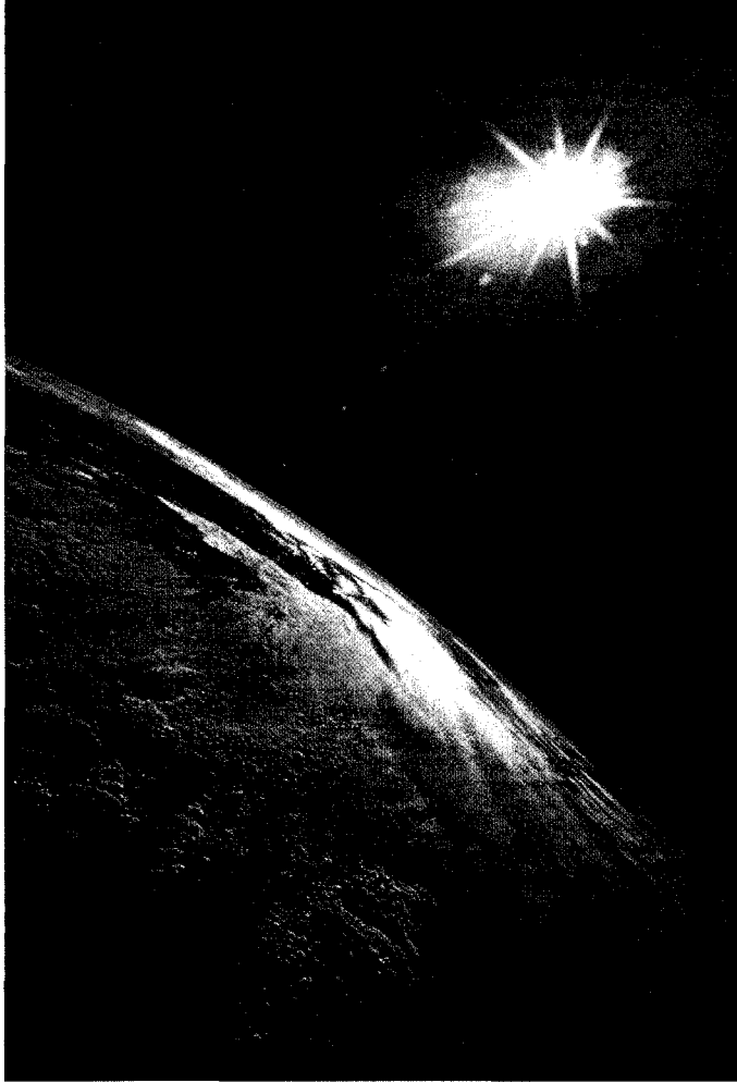
طول الليل والنهار على الأرض مرتبط بثبات سرعة دوران الأرض حول محورها وحول الشمس
